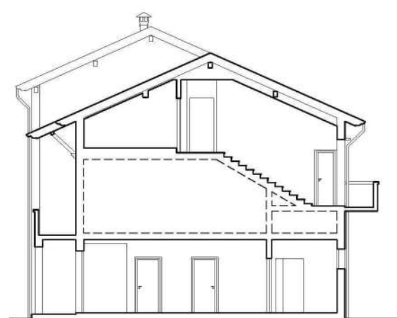
sezione a-a section a-a
