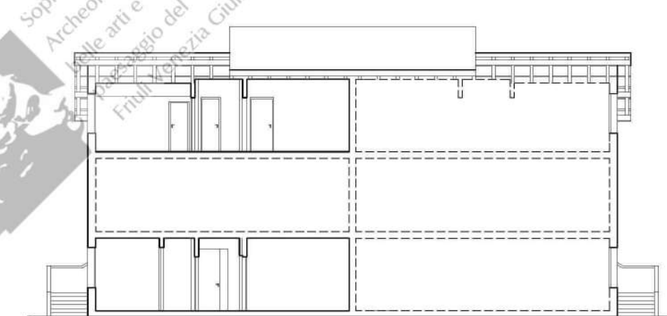
sezione b-b section b-b
