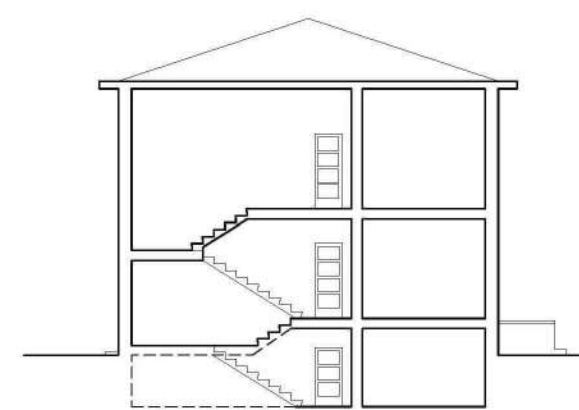
sezione b-b section b-b
