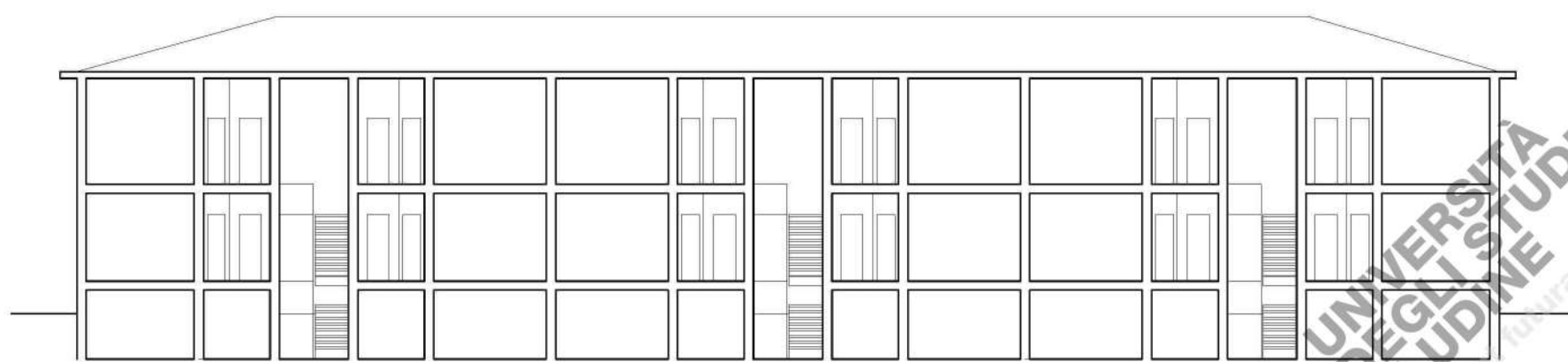
sezione a-a section a-a
