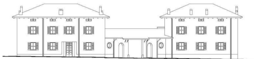
prospetto sud south elevation
